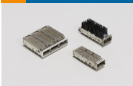
QSFP, QSFP+ & zQSFP+(168)
